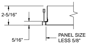
Frame NR (Narrow Regress)
